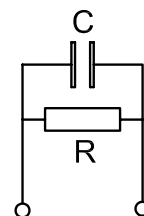
Schemat elektryczny
